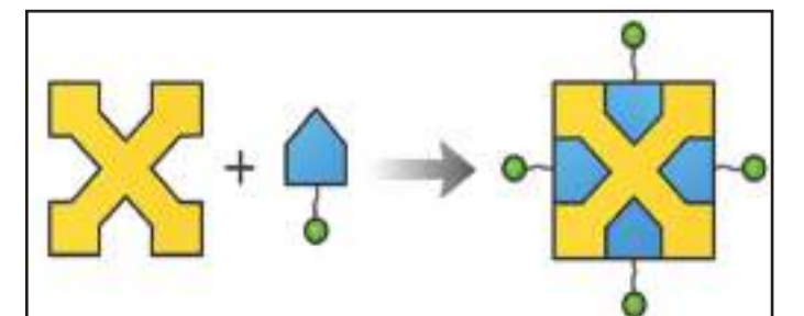
تفاعل الأفيدين (الأصفر) مع البيوتين (الأزرق). جزيء التتبع بنتاديكافلورواوكتانويل موضح بالكور الخضراء
