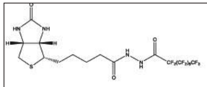
جزيء التتبع بنتاديكافلورواوكتانويل
