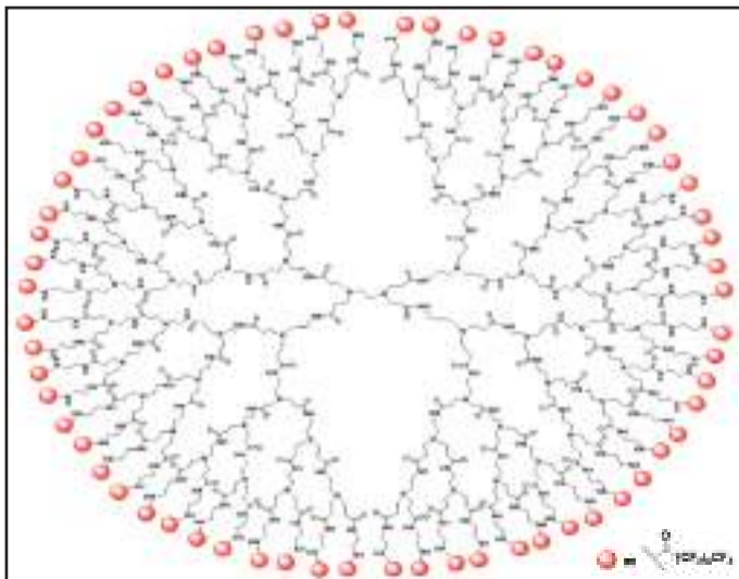
مركب PAMAM المرتبط بجزيء تتبع بنتاديكافلورواوكتانويل (الكور الحمراء)
